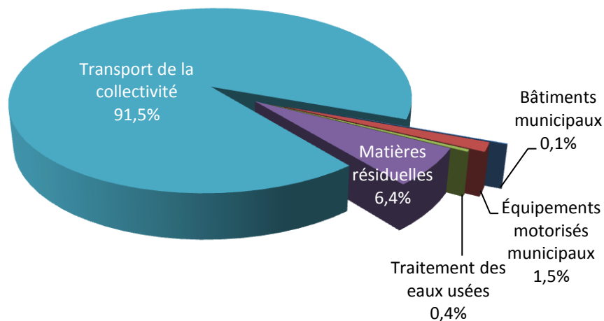
Figure 8.1 : Distribution des émissions globales de GES pour la Ville de Thetford Mines en 2011
