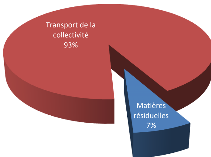
Figure 7.1 : Distribution des émissions de GES de la collectivité pour la Ville de Thetford Mines en 2011
