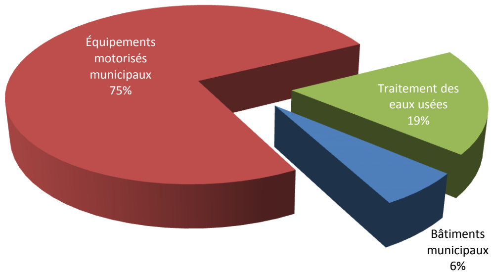
Figure 1 : Distribution des émissions de GES du secteur corporatif pour la Ville de Thetford Mines en 2011
