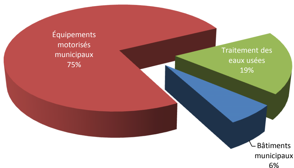
Figure 6.1 : Distribution des émissions corporatives de GES pour la Ville de Thetford Mines en 2011
