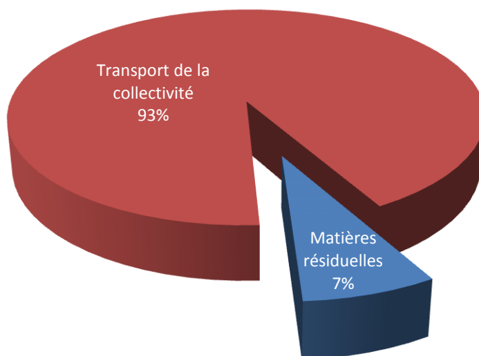
Figure 2 : Distribution des émissions de GES de la collectivité pour la Ville de Thetford Mines en 2011
