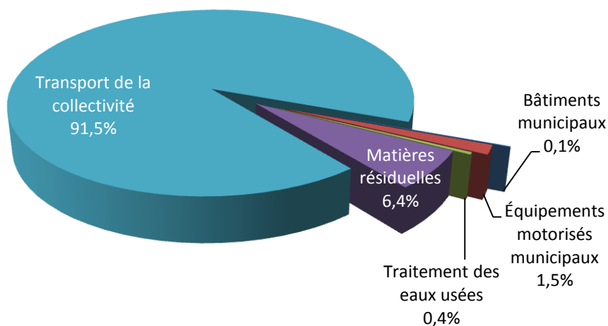
Figure 3 : Distribution des émissions globales de GES pour la Ville de Thetford Mines en 2011
