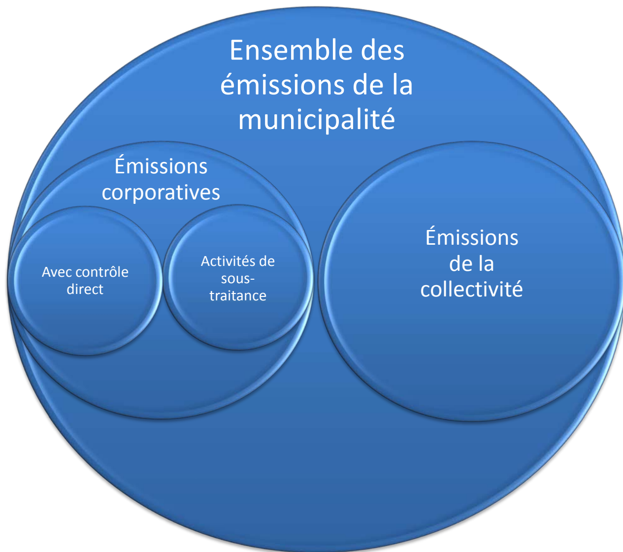
Figure 3.1 : Illustration des secteurs et des champs de l'inventaire GES
