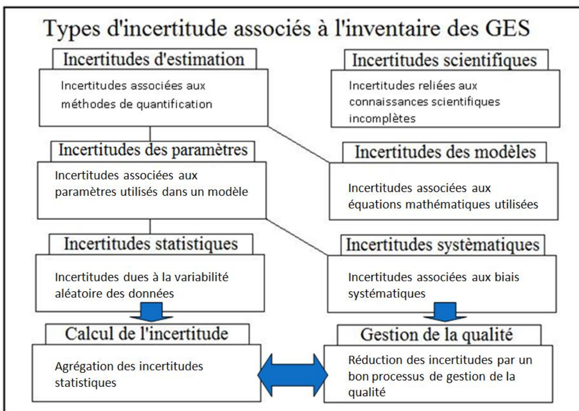
Figure 3.3 : Types d'incertitudes 8
